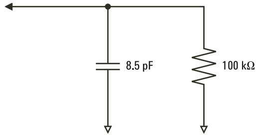
圖 22 DC 和低頻測試棒等效電路
