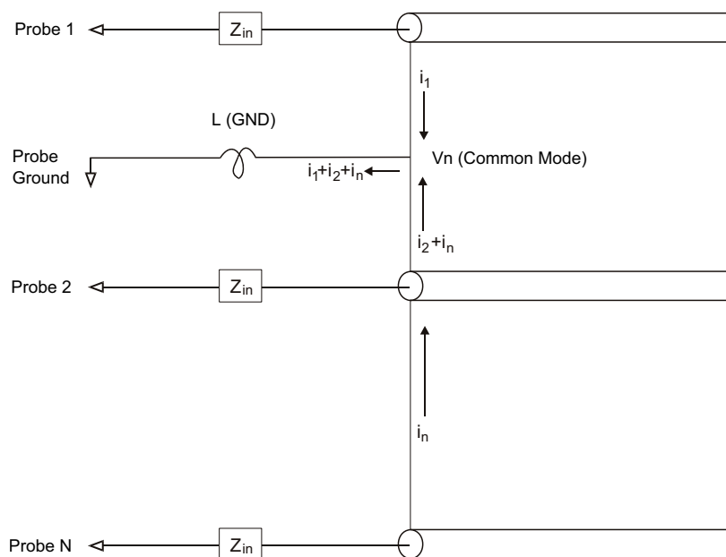
圖 25 共模輸入電壓模型
