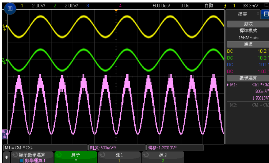
圖 7 通道 1 乘通道 2 範例
