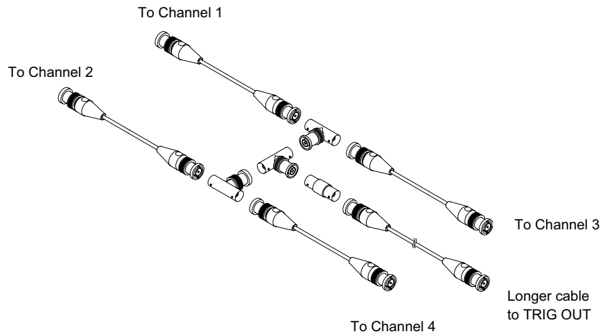
圖 51 4 通道示波器的使用者校準纜線
