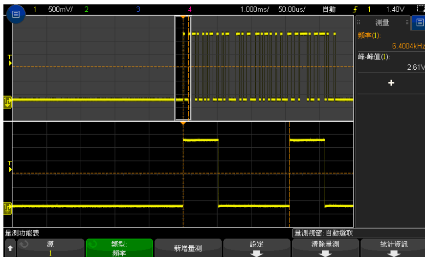
圖 49 區隔頻率量測的事件
