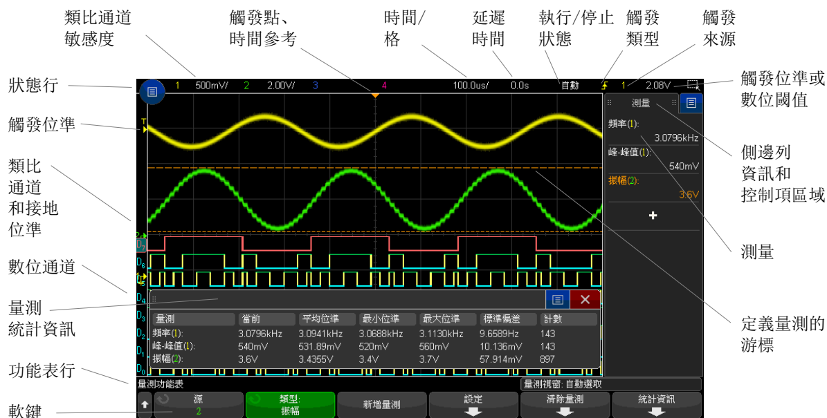
圖 1 解譯示波器顯示
