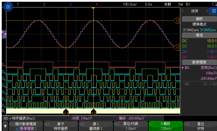
圖 19 邏輯圖匯流排時序範例
