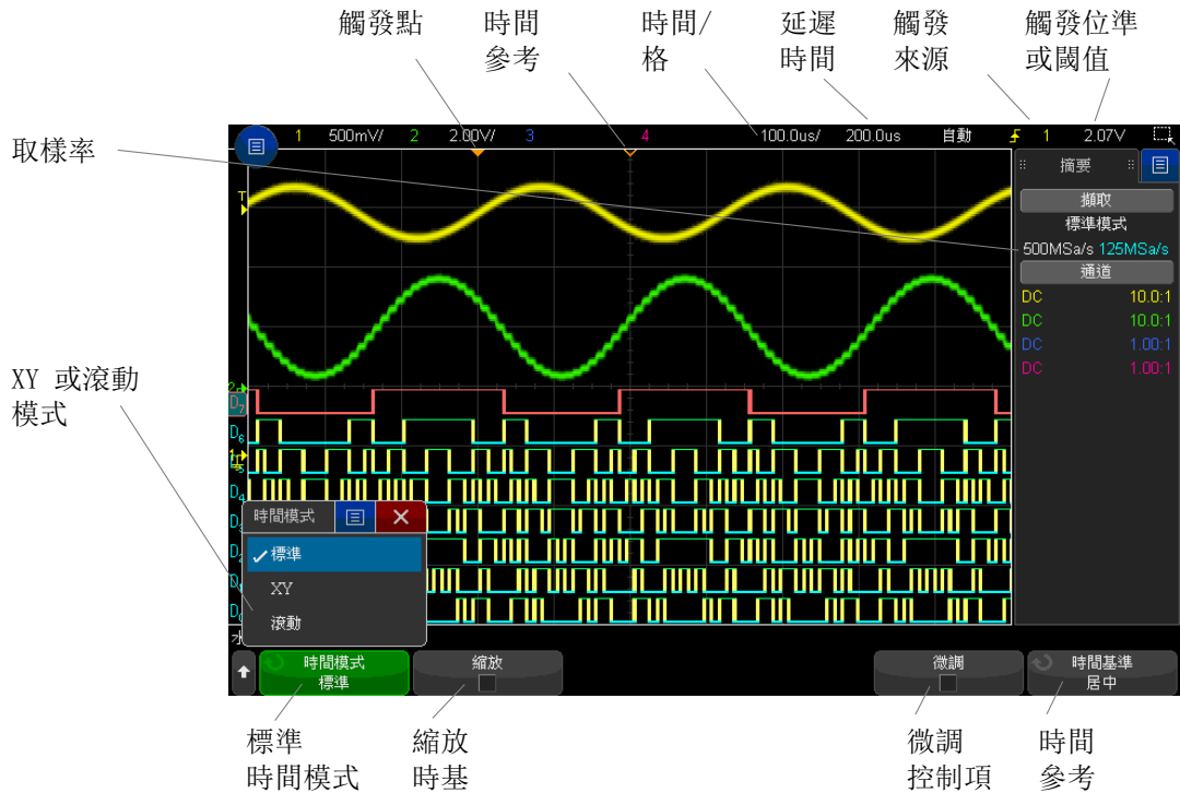
圖 2 「水平設定」功能表
