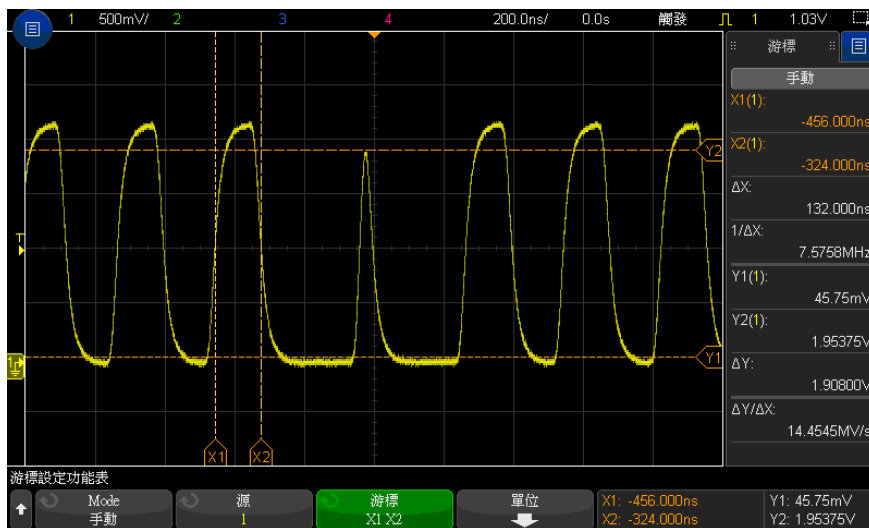
圖 45 一併移動游標以檢查脈波寬度變化
