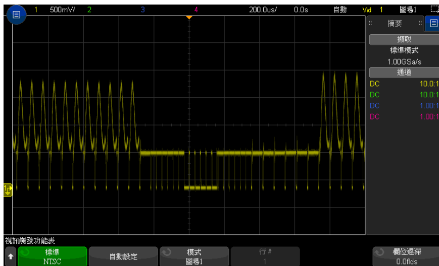
圖 30 針對圖場 1 進行觸發
