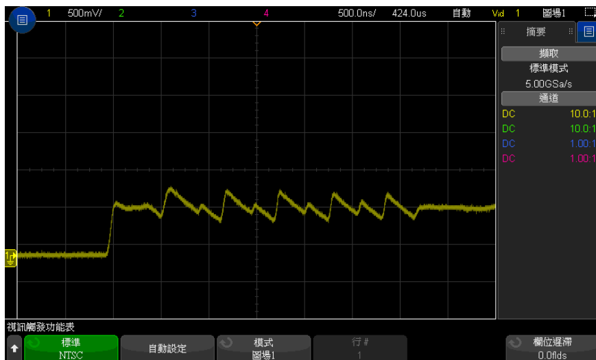
圖 32 針對彩色圖場 1 與彩色圖場 3 進行交替觸發
