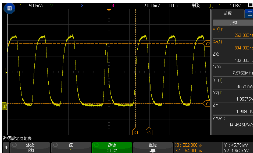
圖 44 使用游標量測脈波寬度
