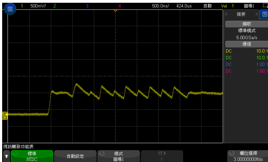
圖 33 使用欄位遲滯同步至彩色圖場 1 或 3 (「圖場 1」模式)
