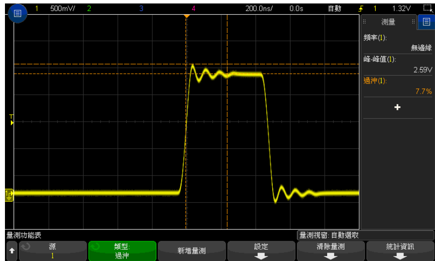
圖 48 自動過沖量測
