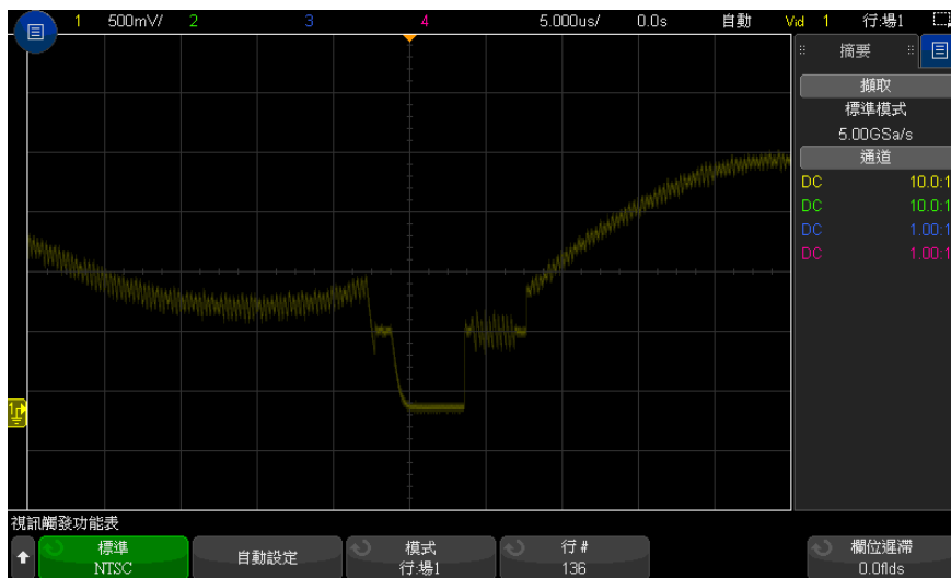
圖 28 範例：針對線 136 進行觸發
