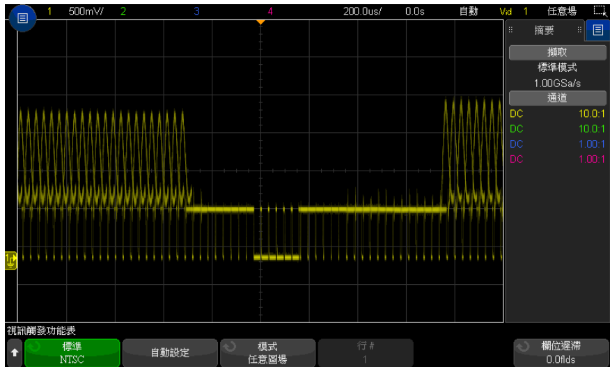
圖 31 針對所有圖場進行觸發
