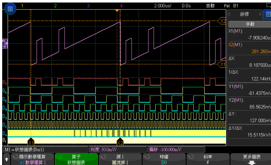
圖 20 邏輯圖匯流排狀態範例
