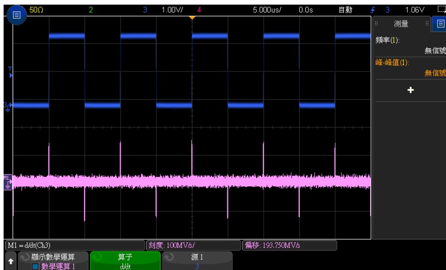
圖 8 微分函數的範例
