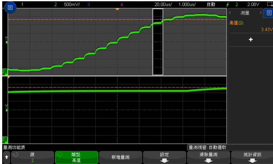
圖 47 區隔頂端量測的區域
