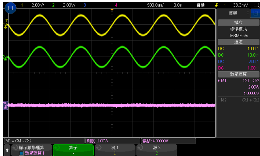
圖 6 通道 1 減通道 2 的範例
