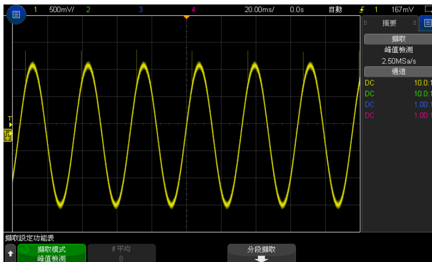
圖 38 具電磁波干擾的正弦，峰值偵測模式
