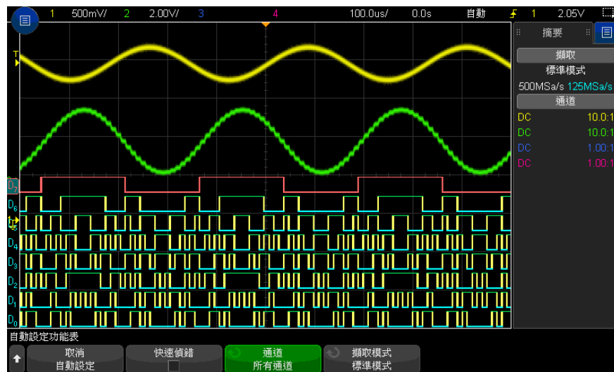
圖 21 範例：數位通道的自動設定（僅限 MSO 機型）
