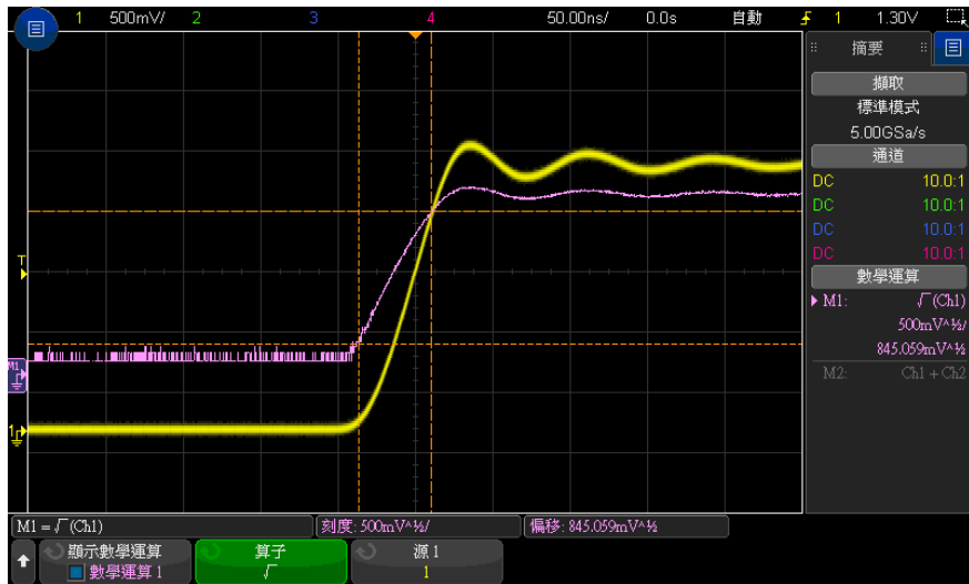
圖 11 \sqrt{\quad} (平方根) 範例
