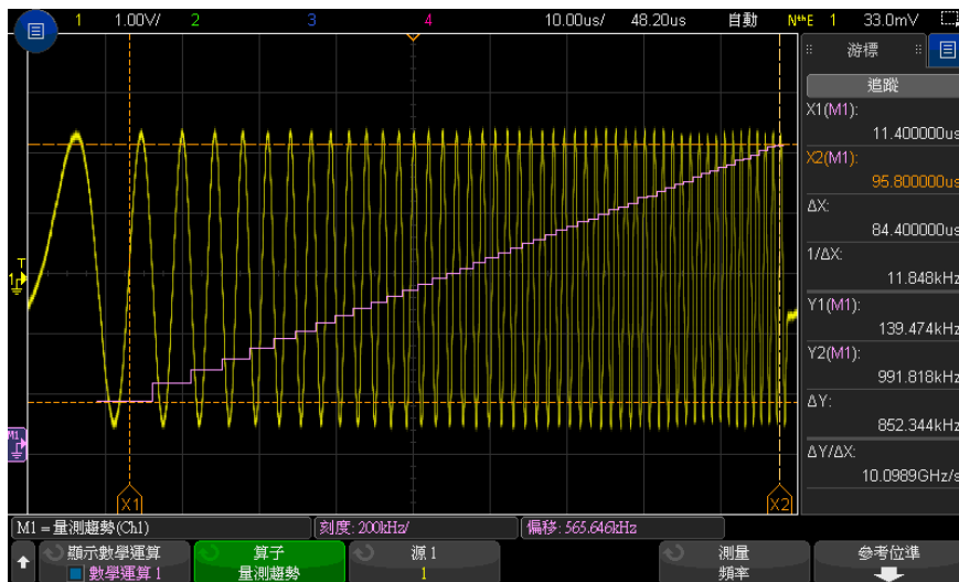
圖 18 量測趨勢範例
