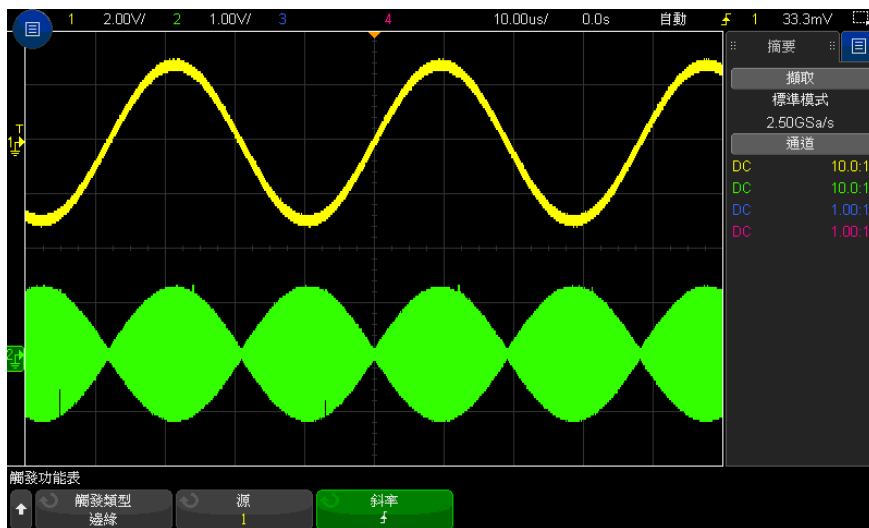
圖 26 以 100% 亮度顯示的幅度調變
