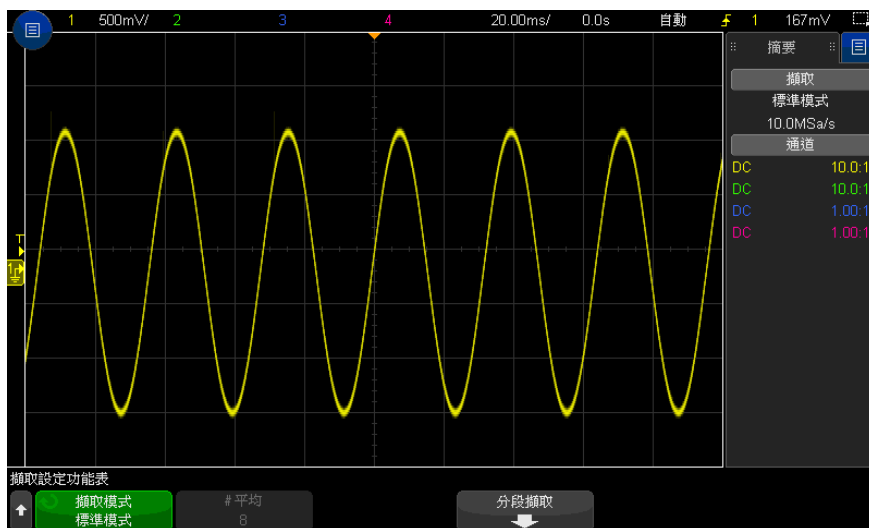
圖 37 具電磁波干擾的正弦，標準模式
