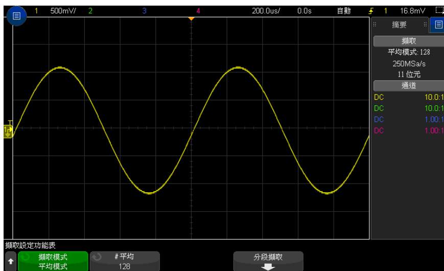
圖 40 對 128 個擷取進行平均以減少隨機雜訊
