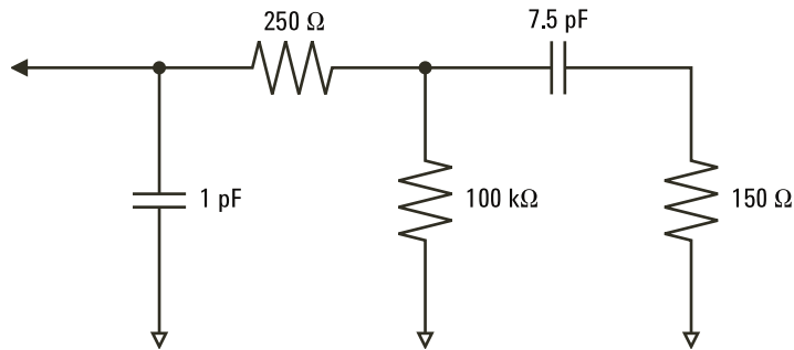
圖 23 高頻測試棒等效電路
