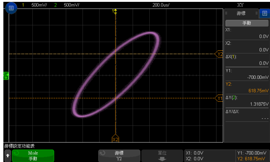
圖 4 相位差量測（自動且使用游標）
