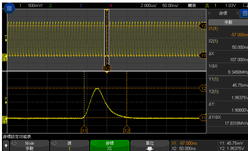
圖 43 游標追蹤縮放視窗
