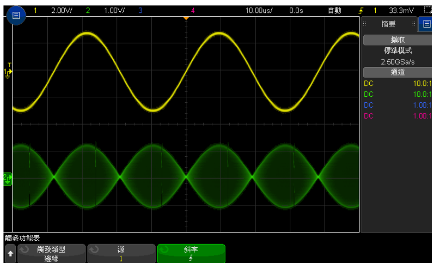
圖 27 以 40% 亮度顯示的幅度調變
