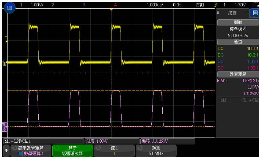
圖 16 低通濾波器範例
