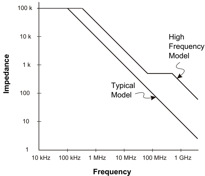
圖 24 兩種測試棒電路模型中阻抗與頻率的關係
