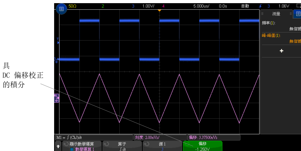
圖 10 具信號偏移的積分
