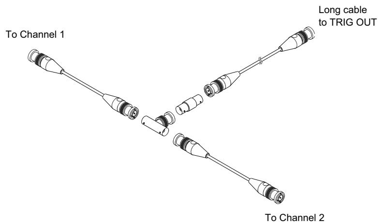
圖 50 2 通道示波器的使用者校準纜線
