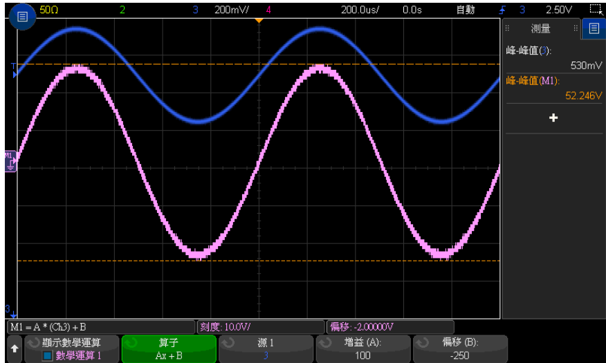
圖 12 Ax + B 範例
