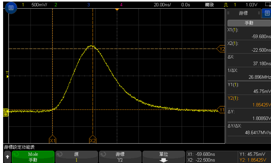
圖 41 用於量測中閾值點以外脈波寬度的游標
