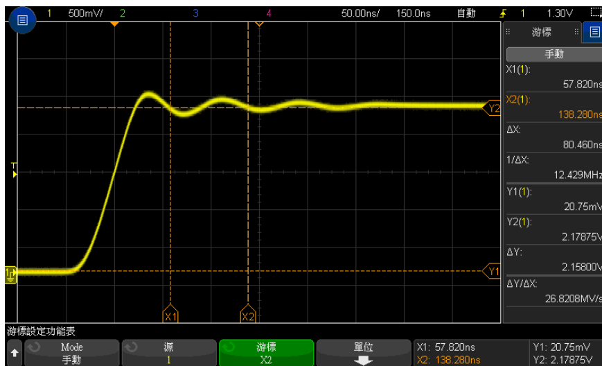
圖 42 量測脈波瞬變頻率的游標
