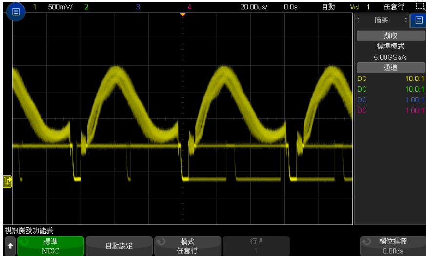
圖 29 針對所有行進行觸發
