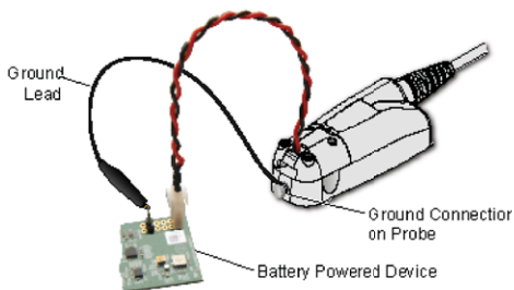
圖 46 使用 N2820A 測試棒在電池供電的裝置上進行量測
