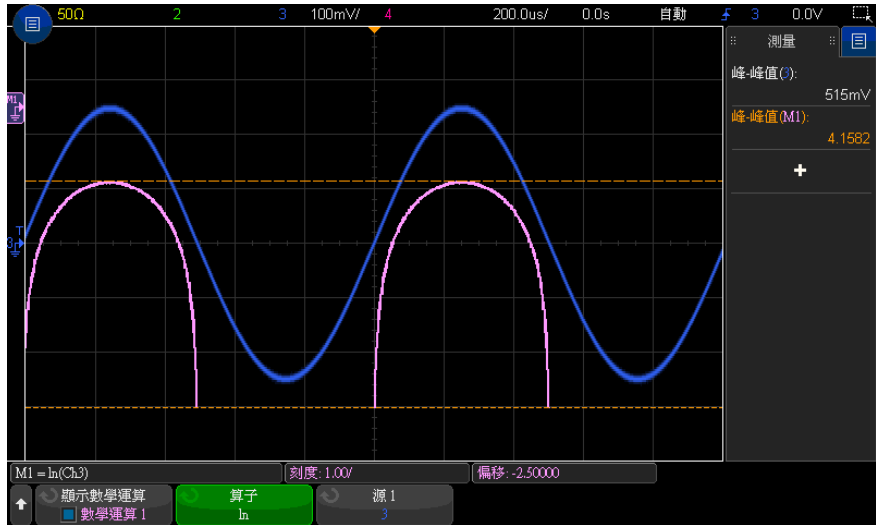
圖 14 自然對數範例
